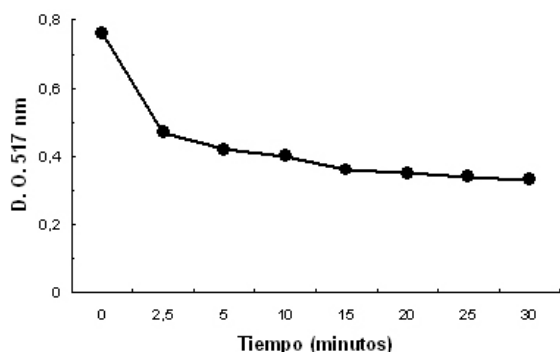
Figura 3. Capacidad depuradora de DPPH de tintura de T. papyriferum utilizando concentraciones de compuestos fenólicos correspondientes a los valores de \text{CD}_{50} e incubados distintos tiempos.
