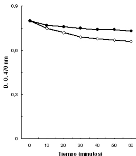
Figura 4. Test de blanqueo de \beta -caroteno frente a dos concentraciones de tintura de T. papyriferum \nabla - 30 \mu\text{g} de compuestos fenólicos/mL - \bullet - 60 \mu\text{g} de compuestos fenólicos/mL.
